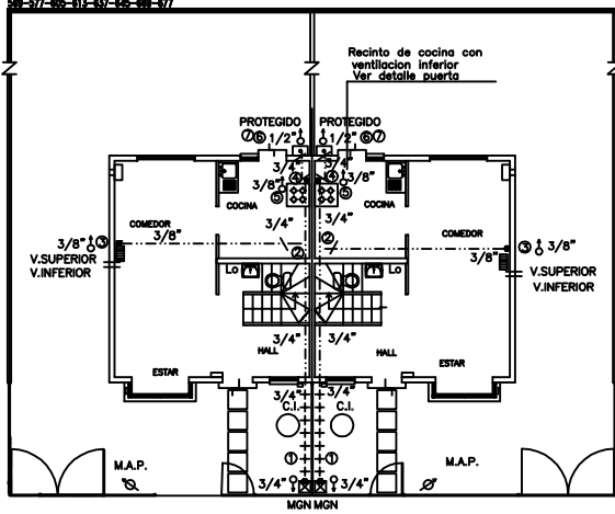
PLANTA PRIMER PISO ESCALA 1/100
