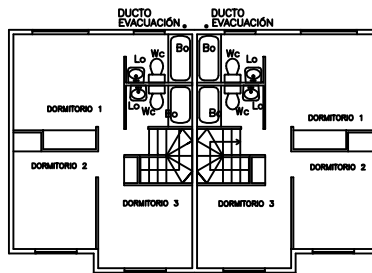
PLANTA SEGUNDO PISO ESCALA 1/100
