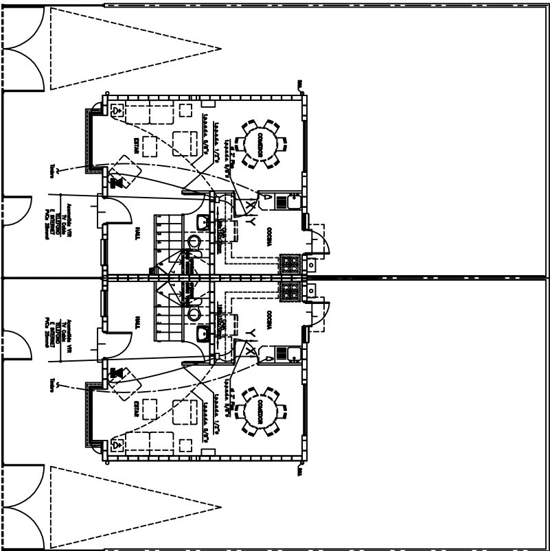
PLANTA PRIMER PISO ESCALA 1:50
