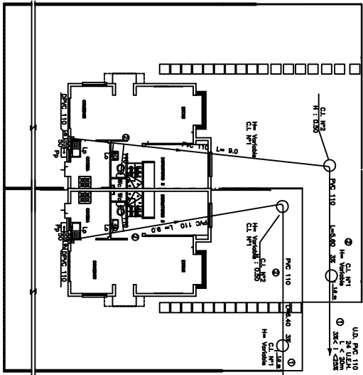
PIANTA 1° PISO Esc. 1100
